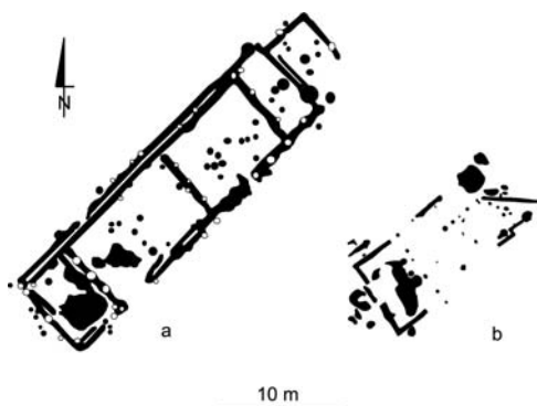
Ryc. 8. Zarysy długich domów datowanych na początek trwania kultury pól popielnicowych; a – Kłodzko-Książek (za Romanow 1971), b – Ruszowice, pow. kłodzki. Rys. J. Baron
